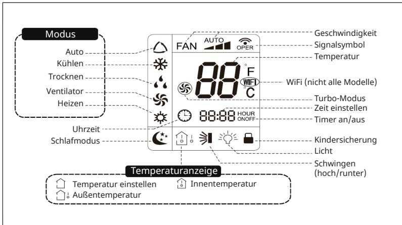
Fernbedienungs-Display
